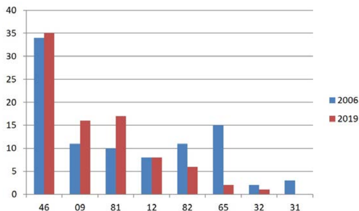
GRAPHE 1 : NOMBRE DE CAVITÉS VISITÉES PAR DÉPARTEMENT EN 2006 ET EN 2019
