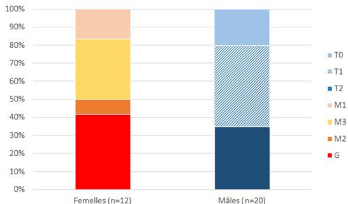
GRAPHE 2 : RÉPARTITION DES DIFFÉRENTS STATUTS SEXUELS EN FONCTION DU SEXE.
