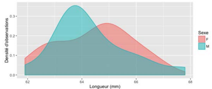
GRAPHE 4: VARIABILITÉ DE LA LONGUEUR DE L'AVANT BRAS EN FONCTION DU SEXE
