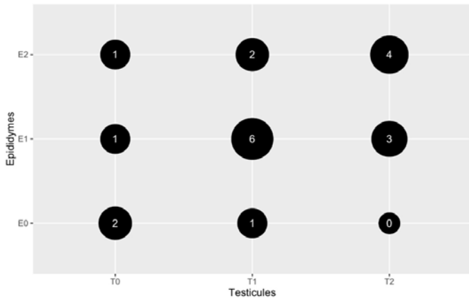
GRAPHE 3: NOMBRE D'INDIVIDU EN FONCTION DES DIFFÉRENTES MODALITÉS DE TAILLES DE TESTICULES ET DE TAILLES D'ÉPIDIDYMES
