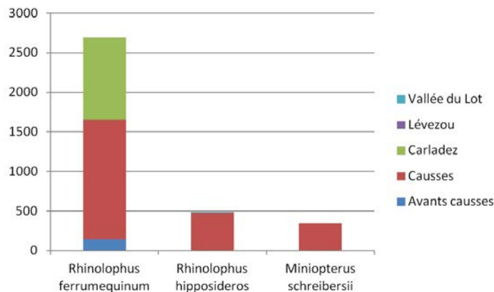
GRAPHE 2: EFFECTIF DES ESPÈCES DE CHAUVES-SOURIS LES PLUS DÉNOMBRÉES PAR L'OBSERVATOIRE DE LA LPO AVEYRON
