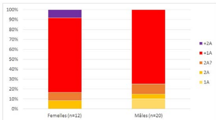
GRAPHE 1 : RÉPARTITION DES DIFFÉRENTES CLASSES D'ÂGE EN FONCTION DU SEXE.
