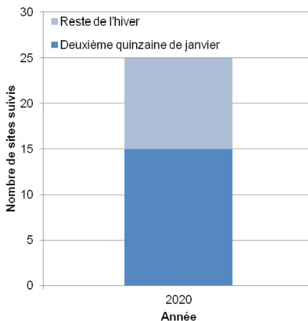
GRAPHE 1: NOMBRE DE SITES D'HIVERNAGE DE CHAUVES-SOURIS SUIVIS
