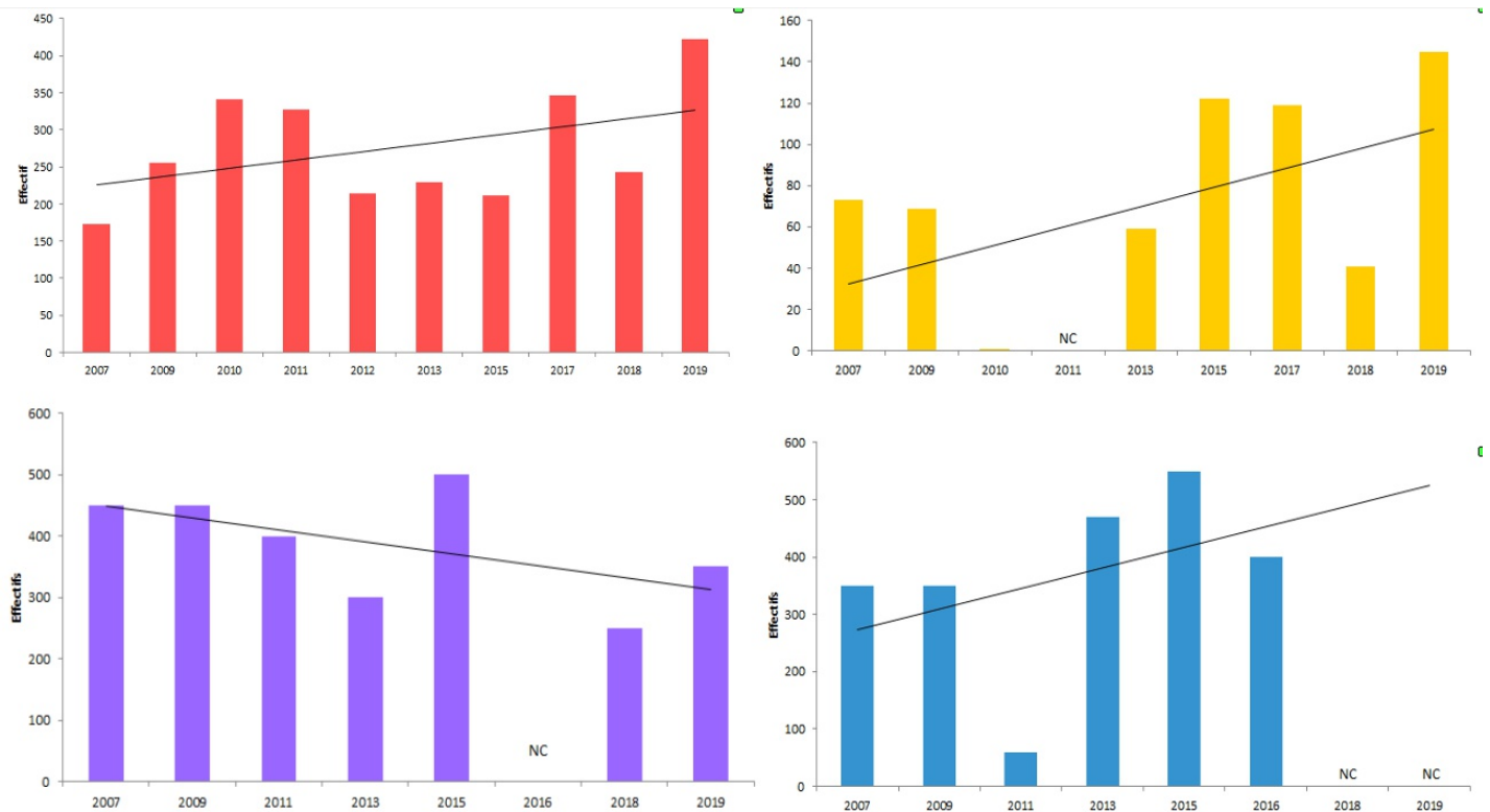
GRAPHE 2 : EVOLUTION DES EFFECTIFS DANS LA GROTTES DU ROY AVEC COURBE DE TENDANCE LINÉAIRE. En haut à gauche : Grand Rhinolophe en hibernation. En haut à droite : Rhinolophe euryale en hibernation. En bas à gauche : Minoptère de Schreibers en transit printanier. En bas à droite : Minoptère de Schreibers en transit automnal.
